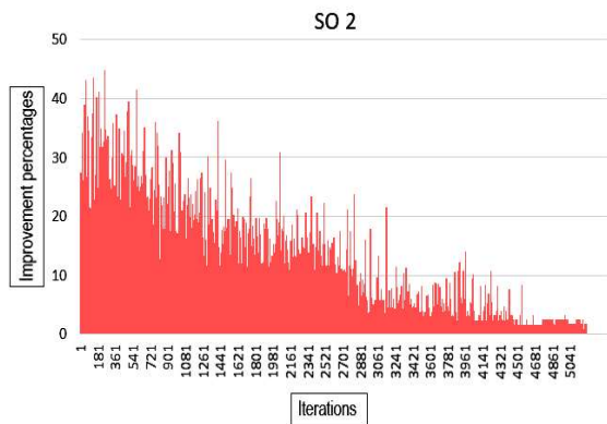
Figure 44: Opérateur de séquençage SO 2.
