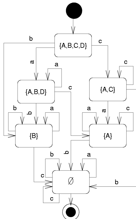
Figure 4 – Diagramme des états de la navigation entre corpus documentaires (notation UML cf. [LAI97], par sélection successive des descripteurs a, b et c (cf. Tab.2).
